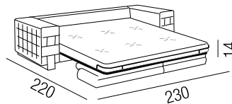
3 POSTI SENZA BRACCIO RETE APERTA 3 SEATER NO ARMREST IN OPEN POSITION 3-Х МЕСТНЫЙ БЕЗ БОКОВИН В РАЗЛОЖЕННОМ ПОЛОЖЕНИИ
